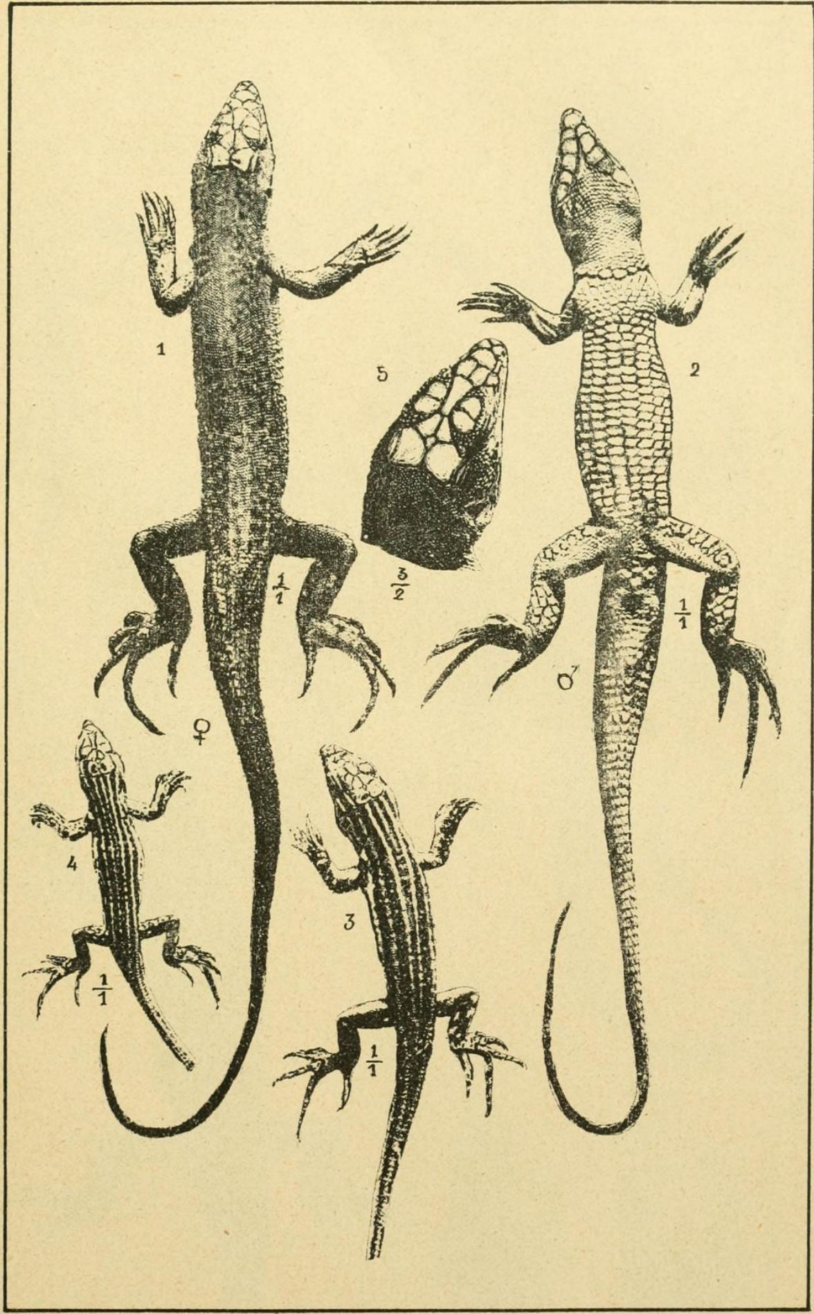
Acanthodactylus Blanci Nob. — Adultes et jeunes. — Hammam-el-Lif (Tunisie)
